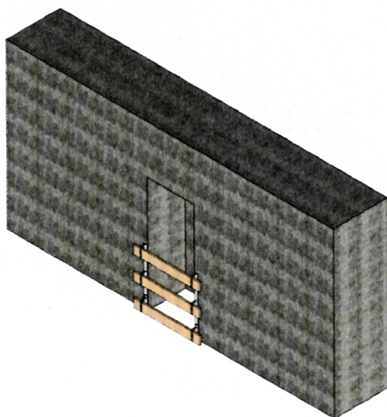
Bild 1: Fahrstuhlschachtabsticherung
